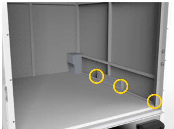
FIGURE 15 : EMLACEMENT DES VIS POUR RETIRER LE PLANCHER
