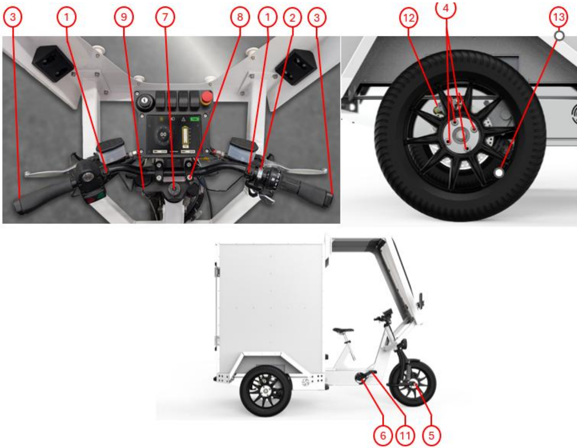
Figure 23 : Emplacement des vis avec les couples fournis
