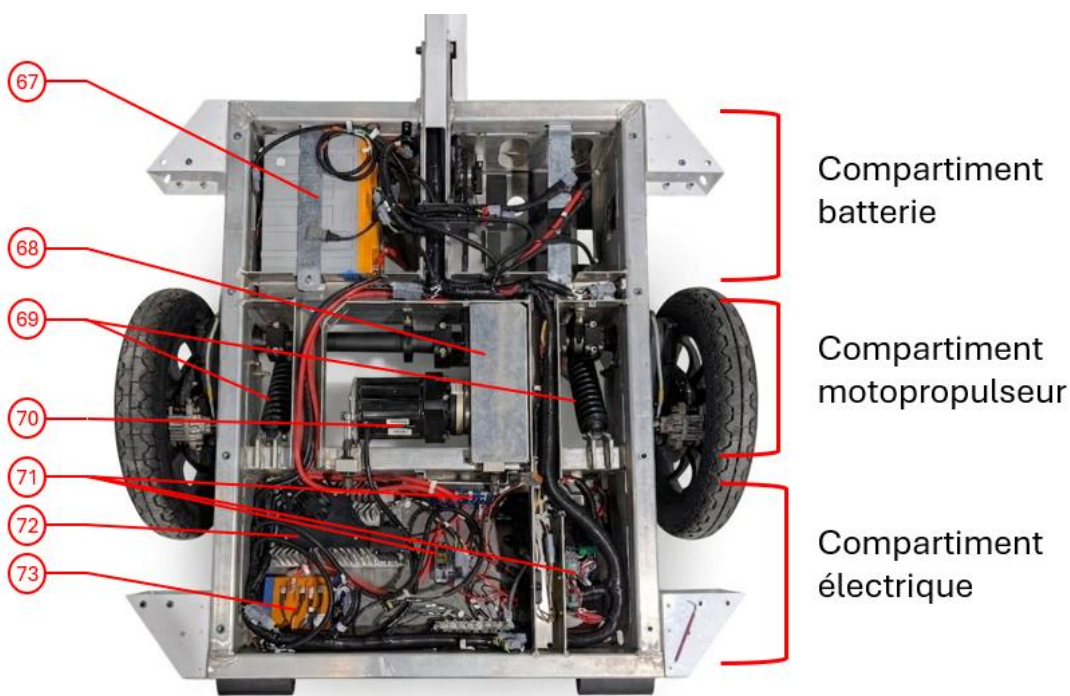
Figure 15 : Emplacement des compartiments
