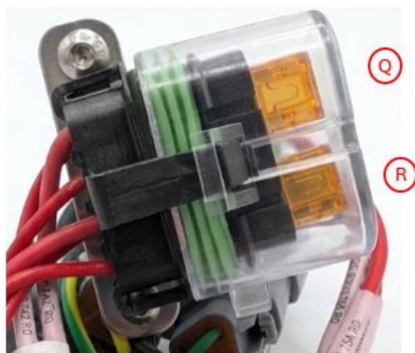
Figure 19 : Boîte à fusible 12V (Écran et système de télémétrie)
